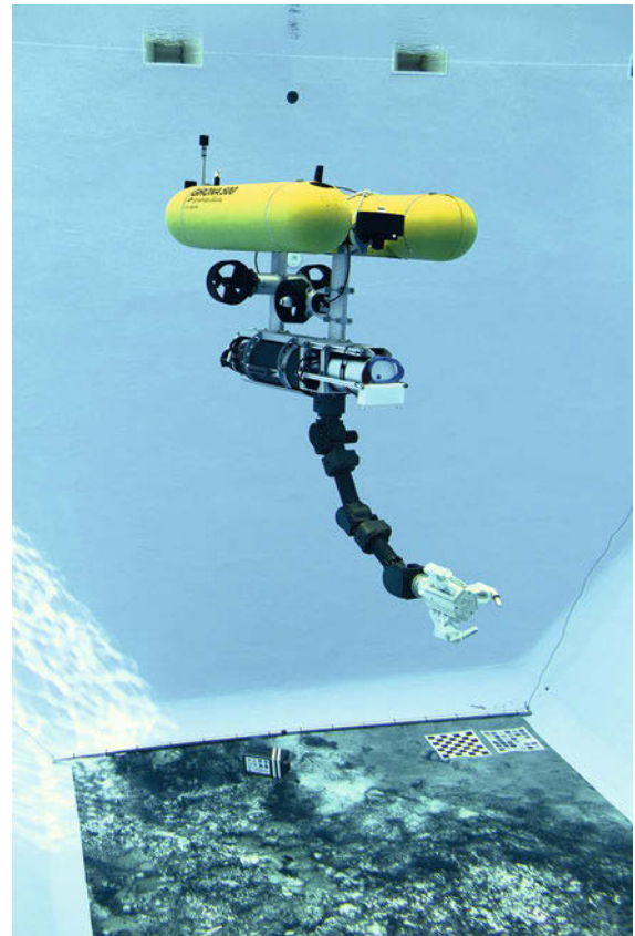
Fig. 25.9 Girona 500 I-AUV
